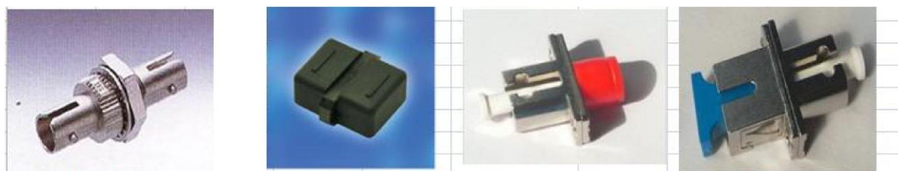
Адаптер AU-b-UbM-srui ST/PC Simplex AD-MP0/SM-SPC1 AD-LC/FC-S AD-LC/SC-S Адаптер MPO Металлический адаптер LC-FC Металлический адаптер LC-SC
